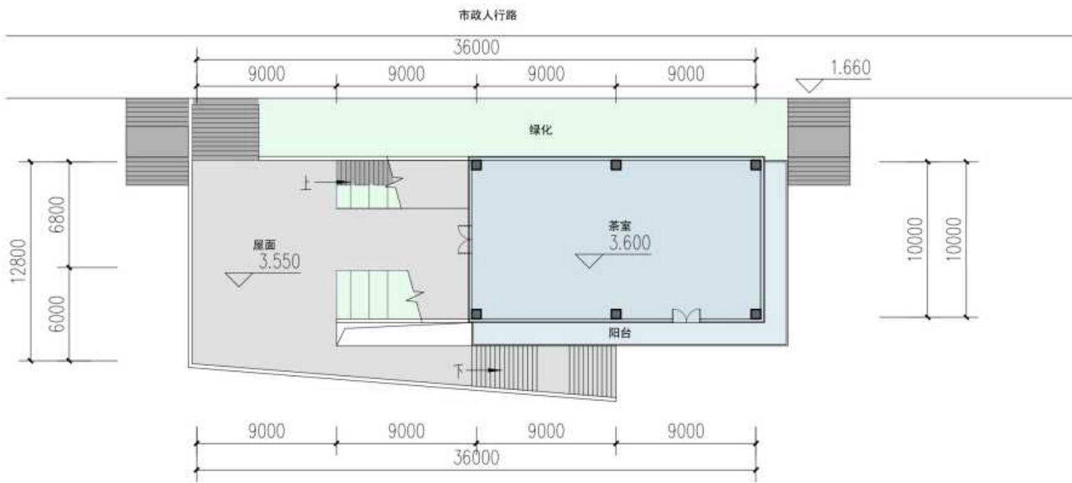
一层平面图
