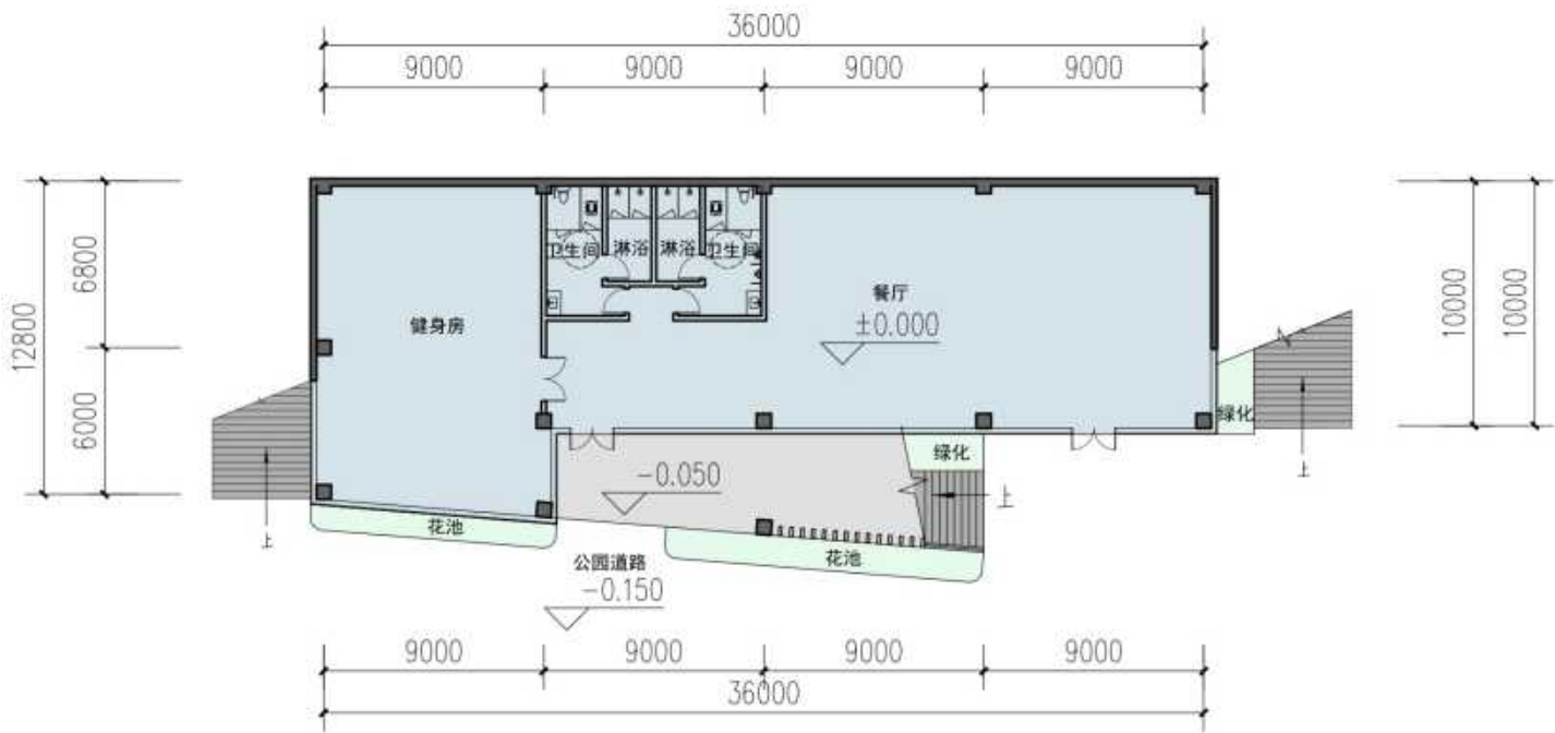
二层平面图
