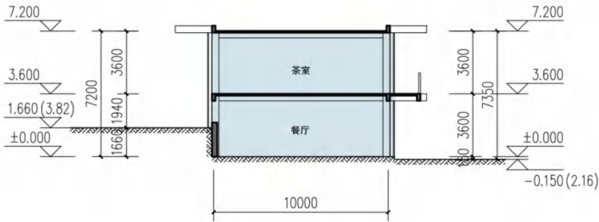
剖面图
