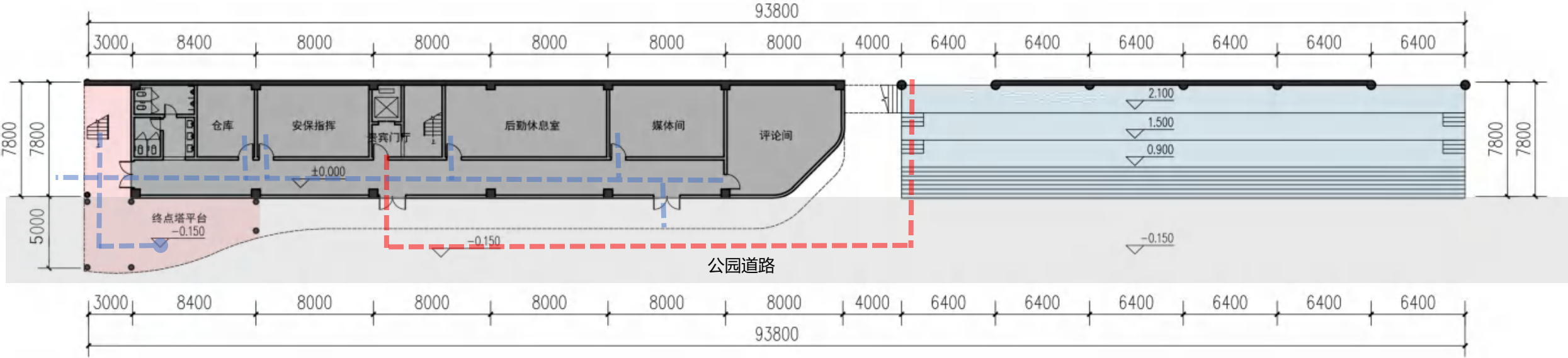
一层平面图
